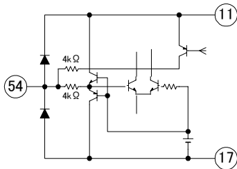
54: BLACK Det
