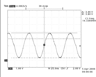
4 IC501-#108
