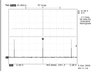
2 V-SYNC
