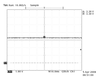
3 IC602-#2
