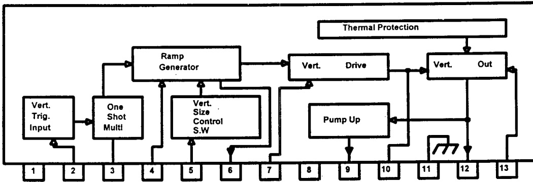
(4) AN614 (IC202)
