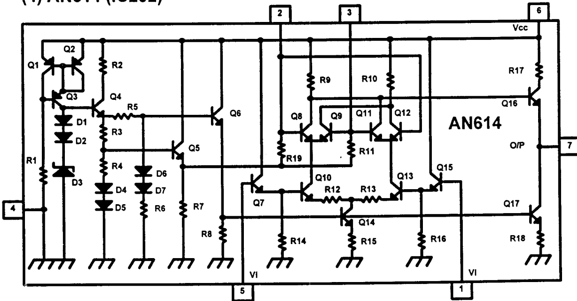
(4) AN614 (IC202)
